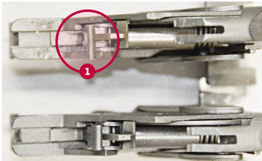
Abbildung 60 Untere Gehäuseteile M 14 und M 1A, oben gut erkennbar der Dauerfeuerhebel des Springfield M 14
