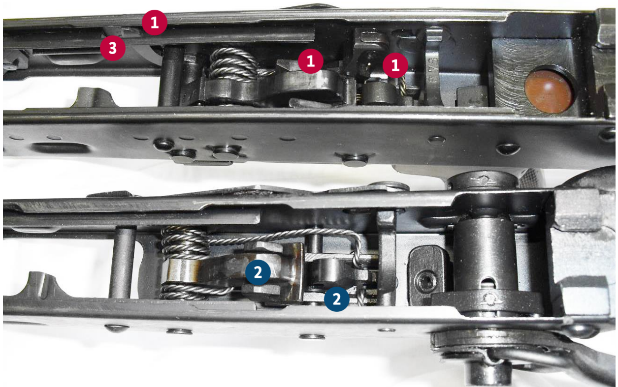
Abbildung 54 Gewehr AK 47, dauerfeuerfähiges Gehäuse oben und halbautomatisches Gehäuse unten.
